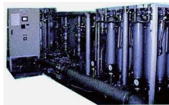
■ 界面活性剤リサイクル装置 半導体加工油、シリコン微粒子等を含んだシリコンウエハ洗浄機用界面活性剤を濾過再利用する装置
